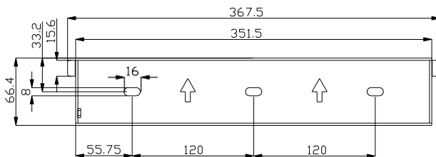
Figura 4.5 Dimensões do painel traseiro de R5-(7K, 7,5K, 8K)-S2-15
