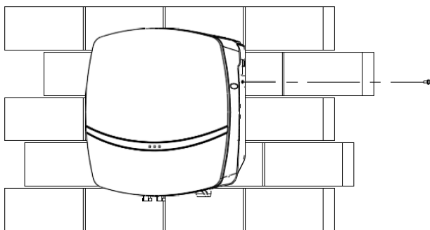
Figura 4.10 Aperte o inversor e o painel suspenso com parafusos.
