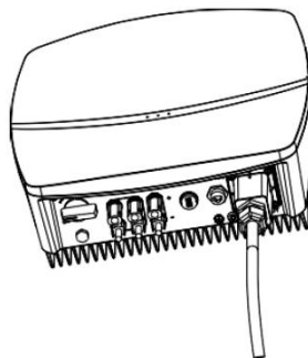
Figura 5.121 Aperte a tampa protetora da interface CA e o trava
