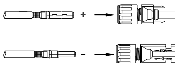
Figura 5.16 Inserindo cabos crimpados nos conectores
