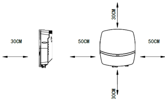
4.2 Posição de Instalação
